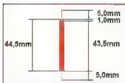
De kortgesloten kwart-golf stub met kwart-golf straler.
